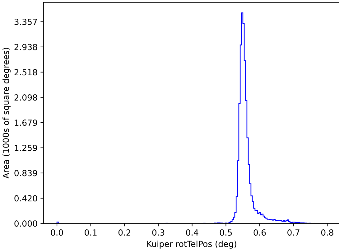
weather_cloudso16v3.5_10yrs y: Kuiper rotTelPos
