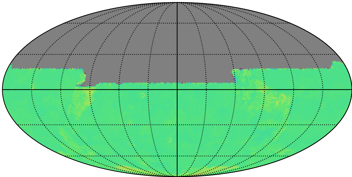
weather_cloudso16v3.5_10yrs y: Kuiper rotTelPos
