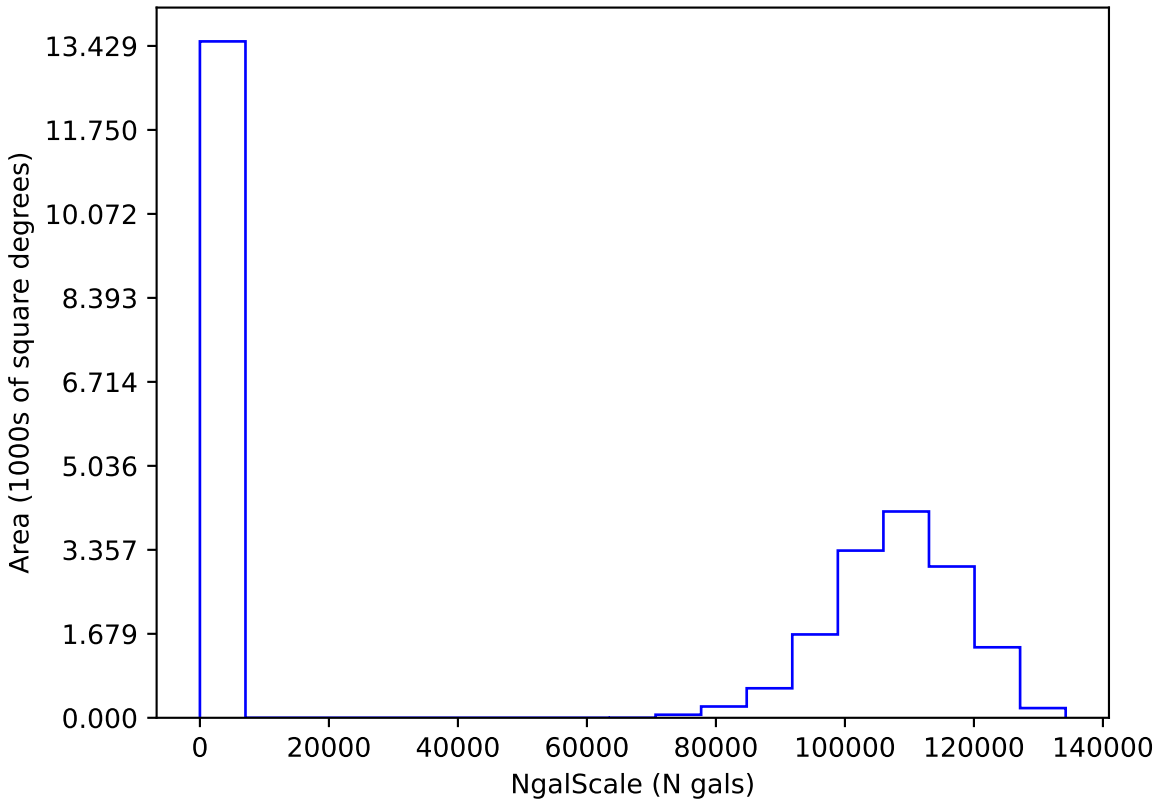
weather_cloudso16v3.5_10yrs i: NgalScale
