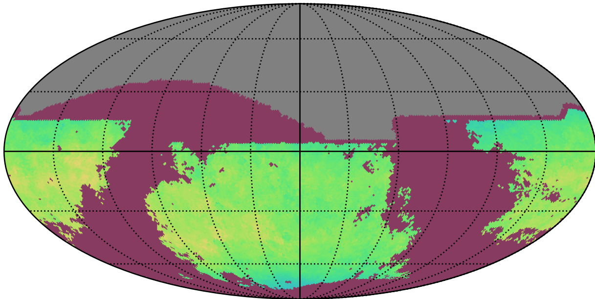
weather_cloudso16v3.5_10yrs i: NgalScale
