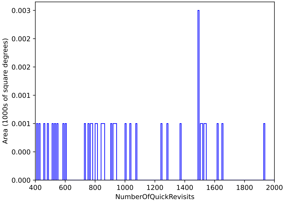
weather_cloudso16v3.5_10yrs : NumberOfQuickRevisits
