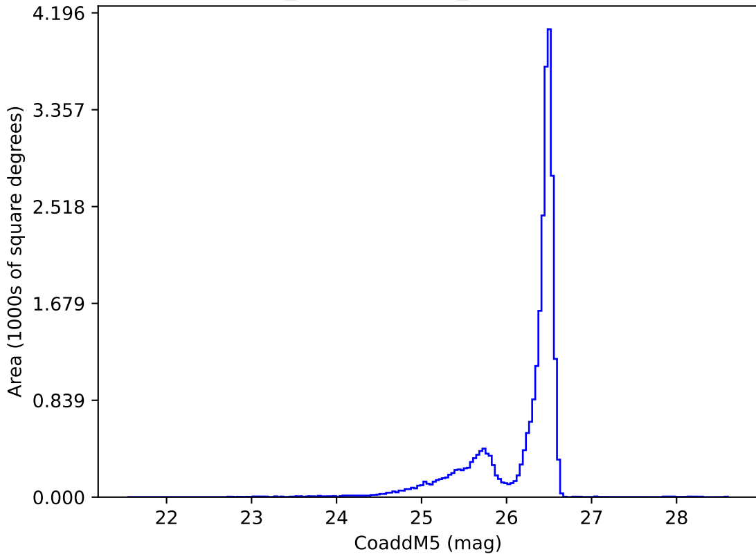
weather_cloudso18v3.5_10yrs i: CoaddM5
