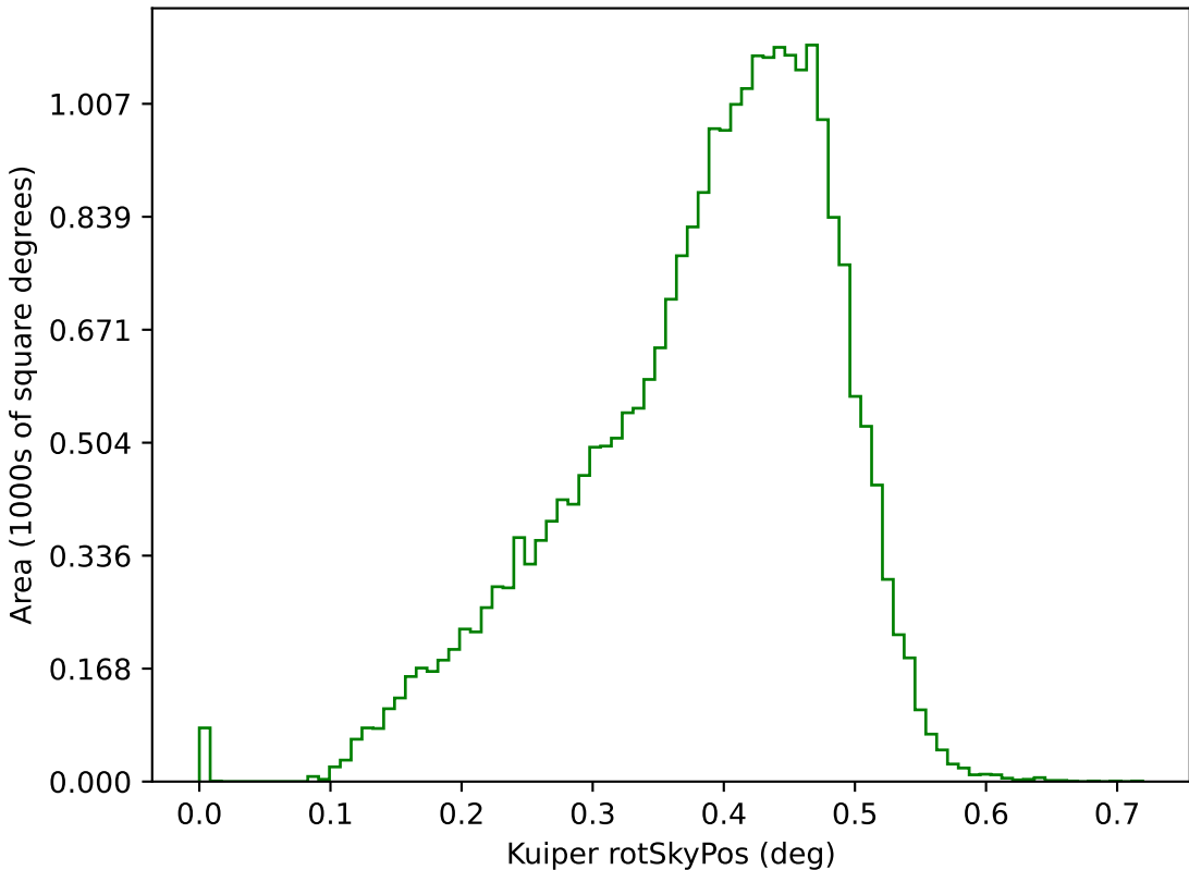
weather_cloudso18v3.5_10yrs g: Kuiper rotSkyPos
