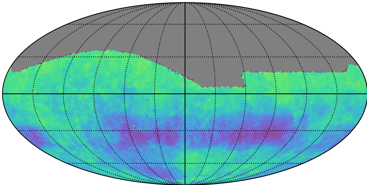
weather_cloudso18v3.5_10yrs g: Kuiper rotSkyPos
