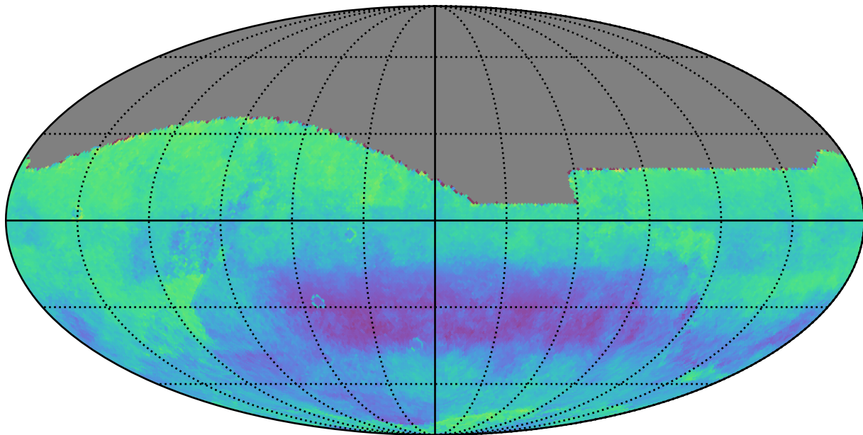
weather_cloudso18v3.5_10yrs i: Kuiper rotSkyPos
