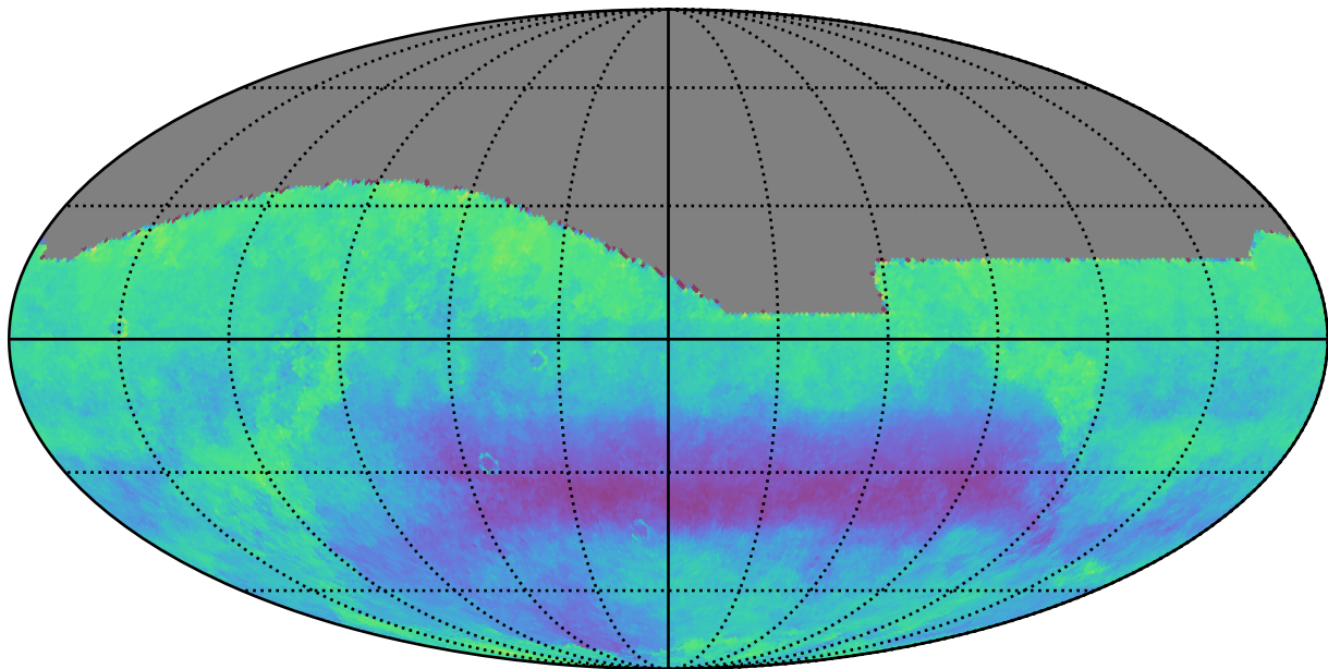
weather_cloudso18v3.5_10yrs r: Kuiper rotSkyPos
