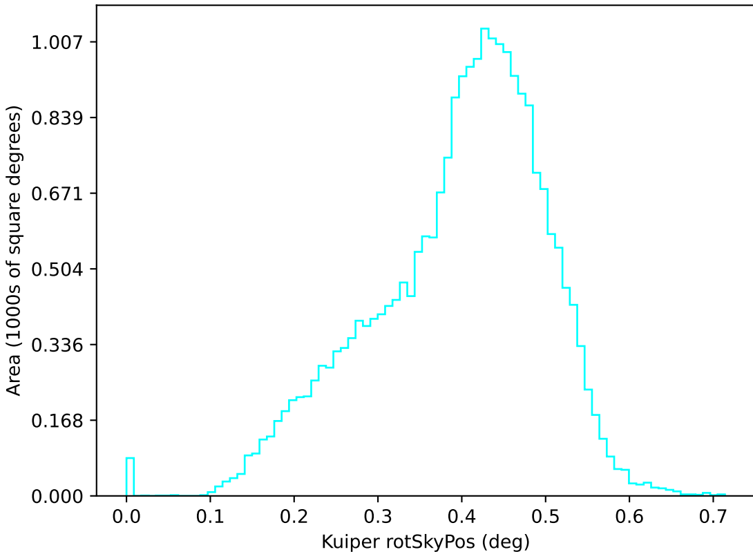
weather_cloudso18v3.5_10yrs u: Kuiper rotSkyPos
