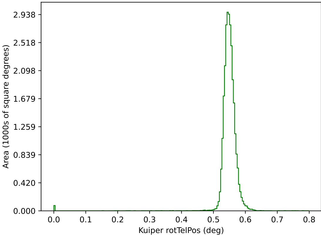
weather_cloudso18v3.5_10yrs g: Kuiper rotTelPos
