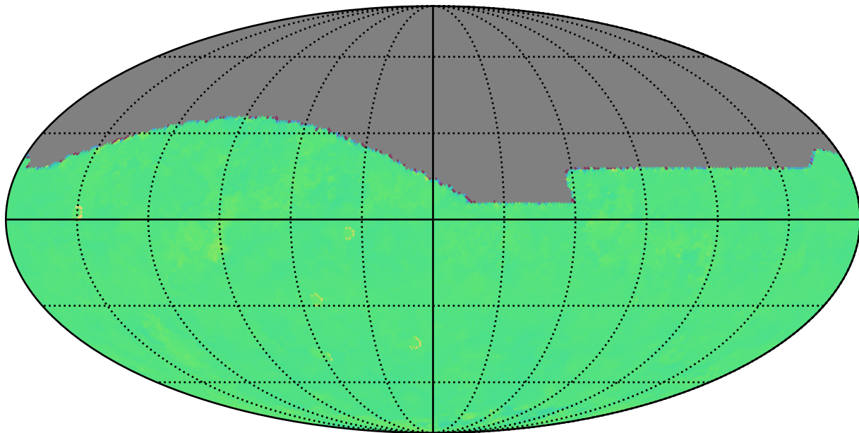
weather_cloudso18v3.5_10yrs i: Kuiper rotTelPos
