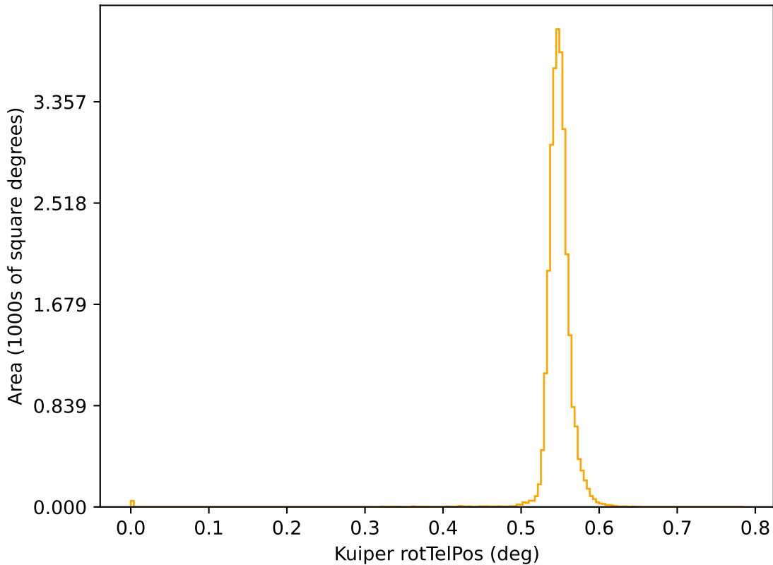
weather_cloudso18v3.5_10yrs r: Kuiper rotTelPos
