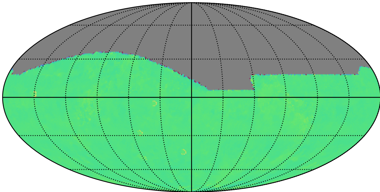
weather_cloudso18v3.5_10yrs r: Kuiper rotTelPos
