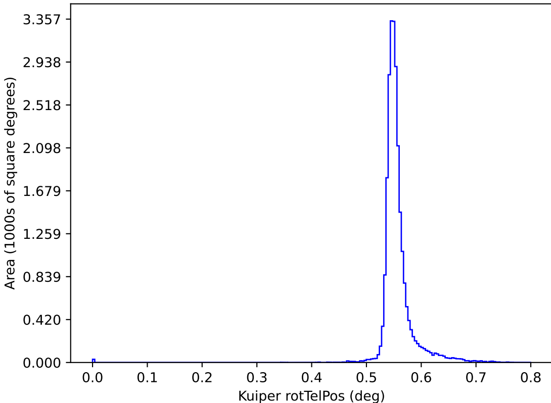
weather_cloudso18v3.5_10yrs y: Kuiper rotTelPos
