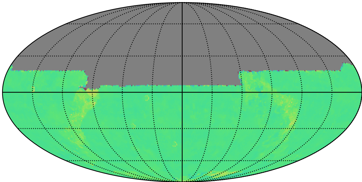
weather_cloudso18v3.5_10yrs y: Kuiper rotTelPos
