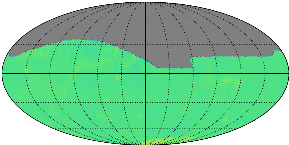
weather_cloudso18v3.5_10yrs z: Kuiper rotTelPos
