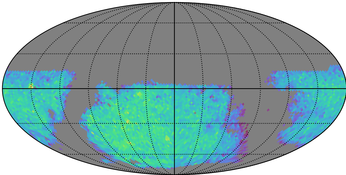
weather_cloudso18v3.5_10yrs gi: LVDwarfs
