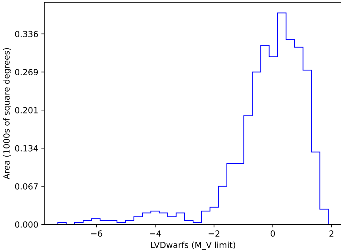
weather_cloudso18v3.5_10yrs gi SCP: LVDwarfs
