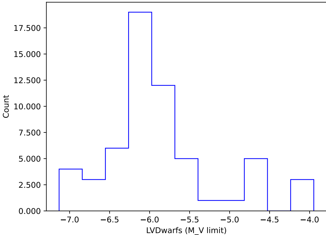
weather_cloudso18v3.5_10yrs gi: LVDwarfs
