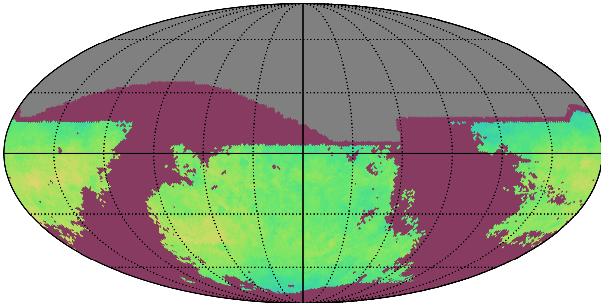
weather_cloudso18v3.5_10yrs i: NgalScale
