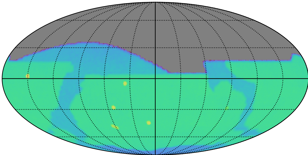
weather_cloudso18v3.5_10yrs i: SurfaceBrightLimit
