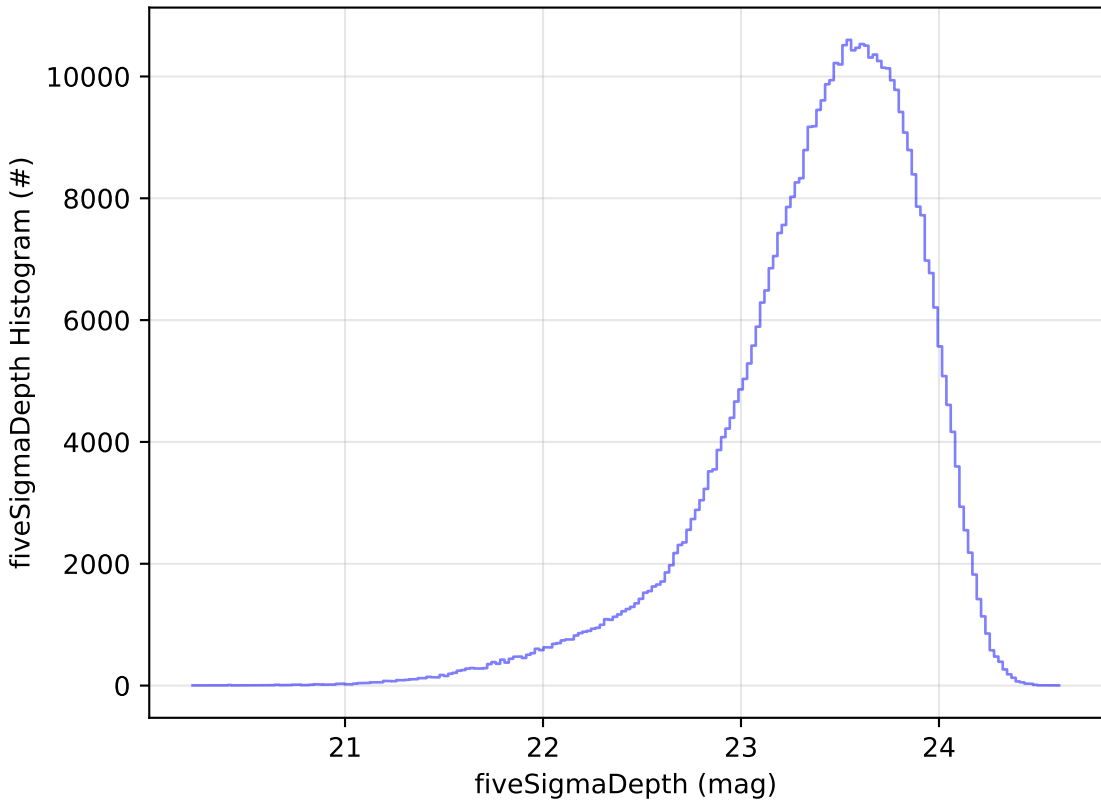
weather_cloudso18v3.5_10yrs i: fiveSigmaDepth Histogram
