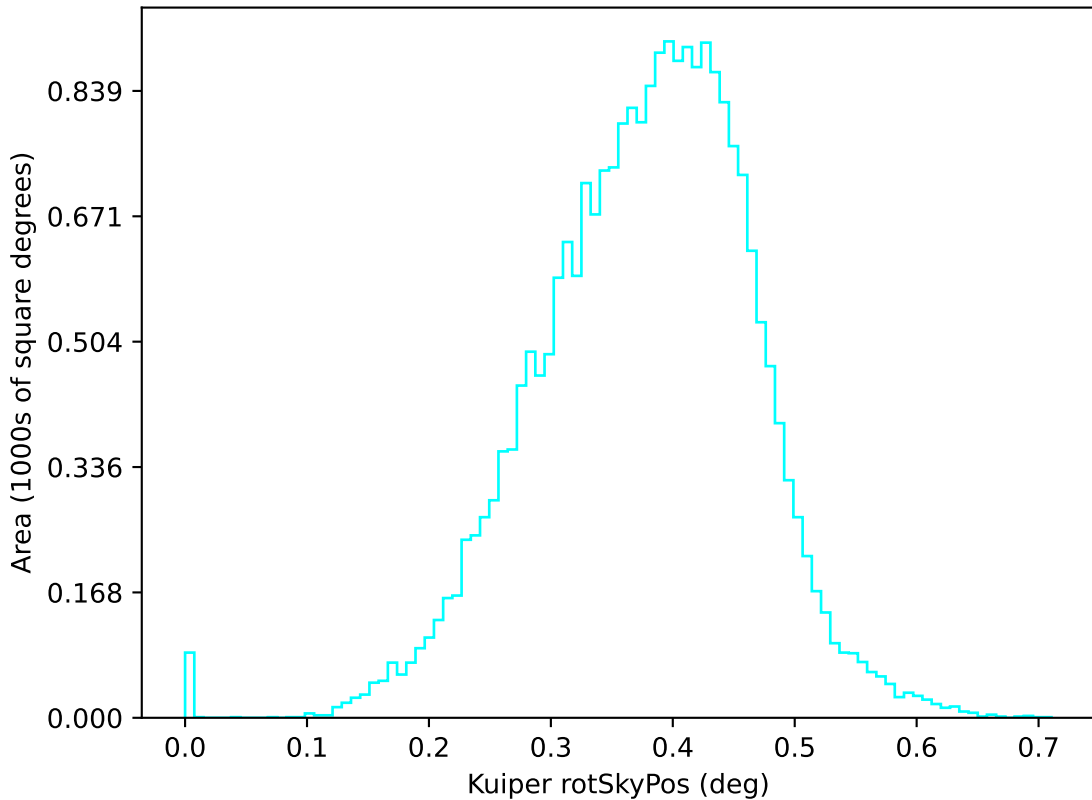
weather_cloudso1v3.5_10yrs u: Kuiper rotSkyPos
