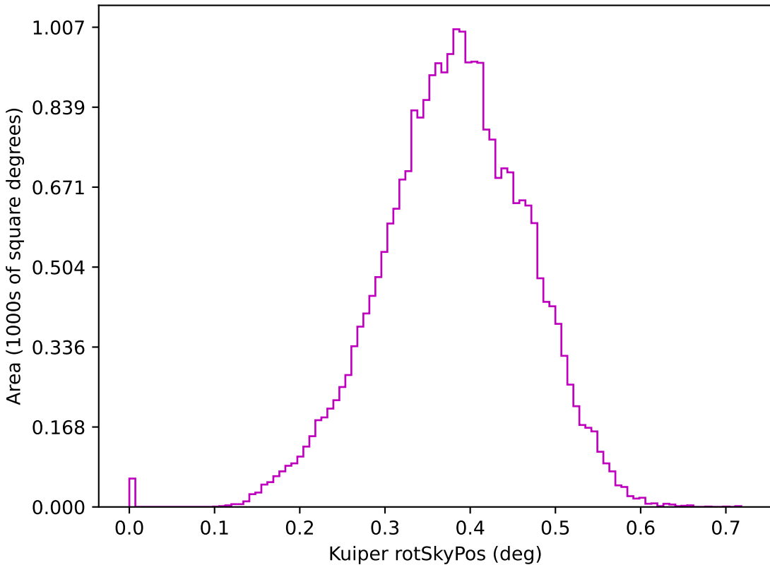
weather_cloudso1v3.5_10yrs z: Kuiper rotSkyPos
