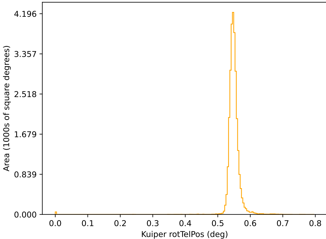
weather_cloudso1v3.5_10yrs r: Kuiper rotTelPos
