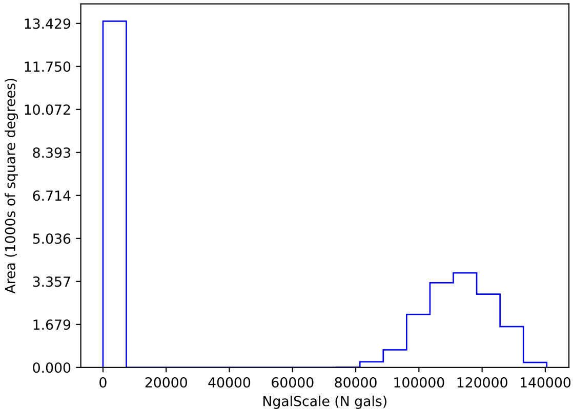
weather_cloudso1v3.5_10yrs i: NgalScale
