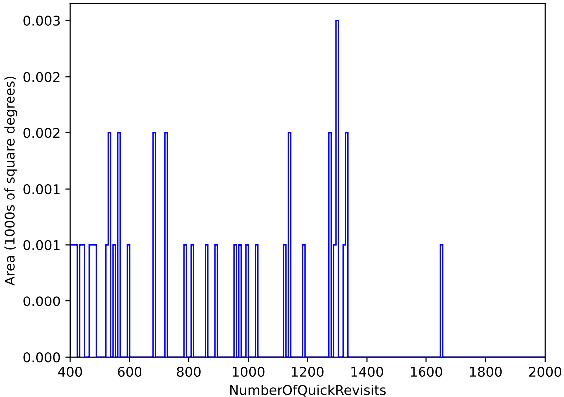
weather_cloudso1v3.5_10yrs : NumberOfQuickRevisits
