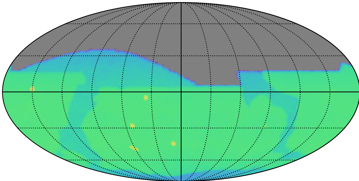
weather_cloudso2v3.5_10yrs i: CoaddM5
