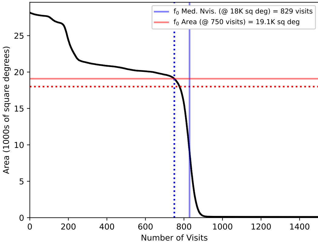
weather_cloudso2v3.5_10yrs : f0
