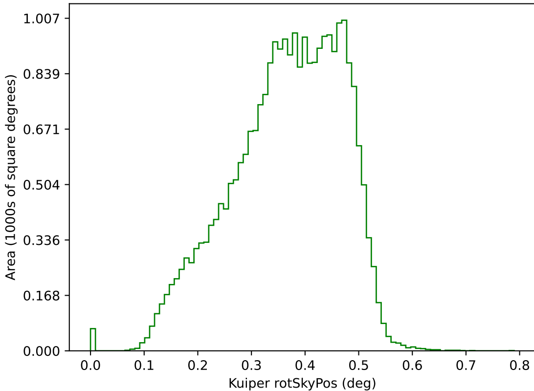
weather_cloudso2v3.5_10yrs g: Kuiper rotSkyPos
