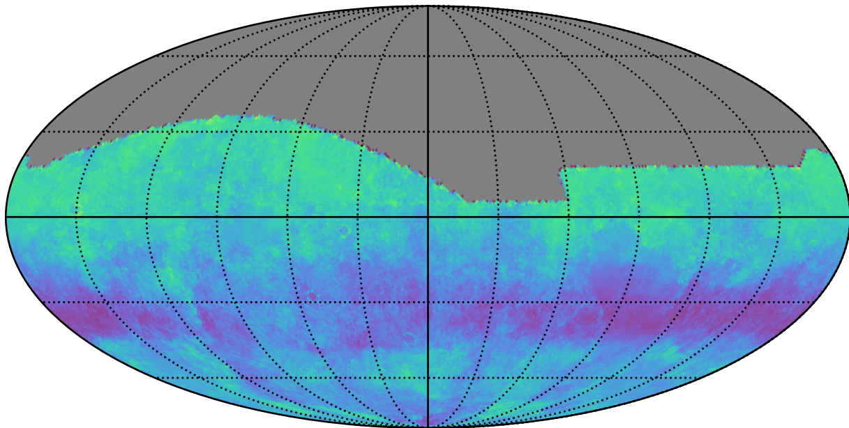
weather_cloudso2v3.5_10yrs g: Kuiper rotSkyPos
