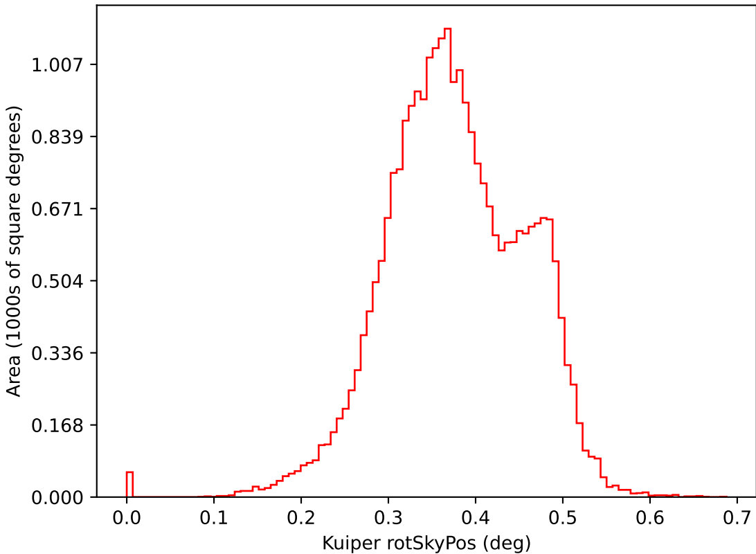
weather_cloudso2v3.5_10yrs i: Kuiper rotSkyPos
