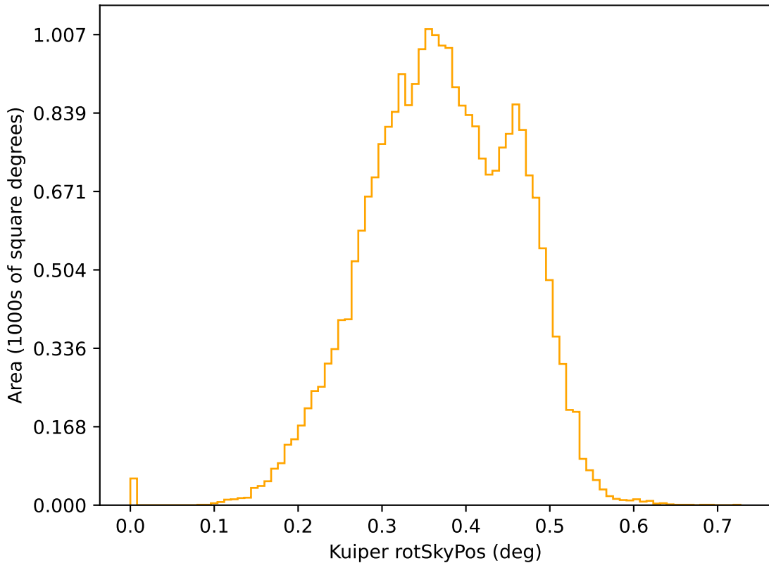
weather_cloudso2v3.5_10yrs r: Kuiper rotSkyPos
