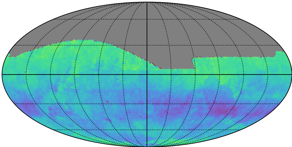
weather_cloudso2v3.5_10yrs r: Kuiper rotSkyPos
