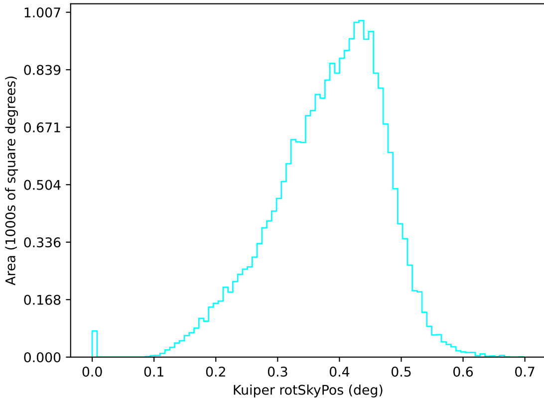
weather_cloudso2v3.5_10yrs u: Kuiper rotSkyPos
