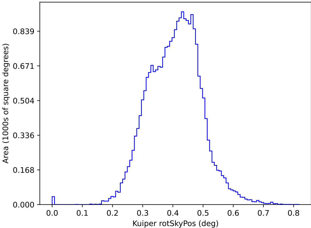
weather_cloudso2v3.5_10yrs y: Kuiper rotSkyPos
