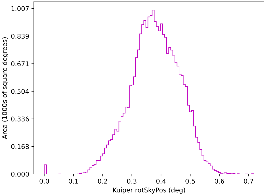
weather_cloudso2v3.5_10yrs z: Kuiper rotSkyPos
