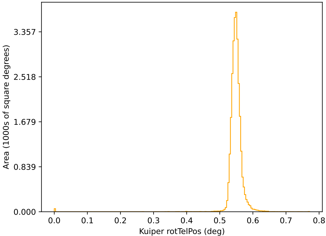
weather_cloudso2v3.5_10yrs r: Kuiper rotTelPos
