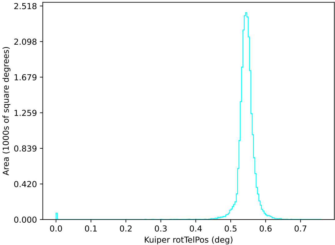
weather_cloudso2v3.5_10yrs u: Kuiper rotTelPos
