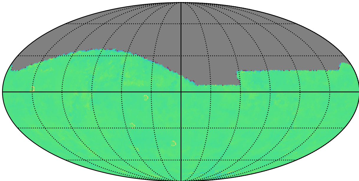
weather_cloudso2v3.5_10yrs z: Kuiper rotTelPos
