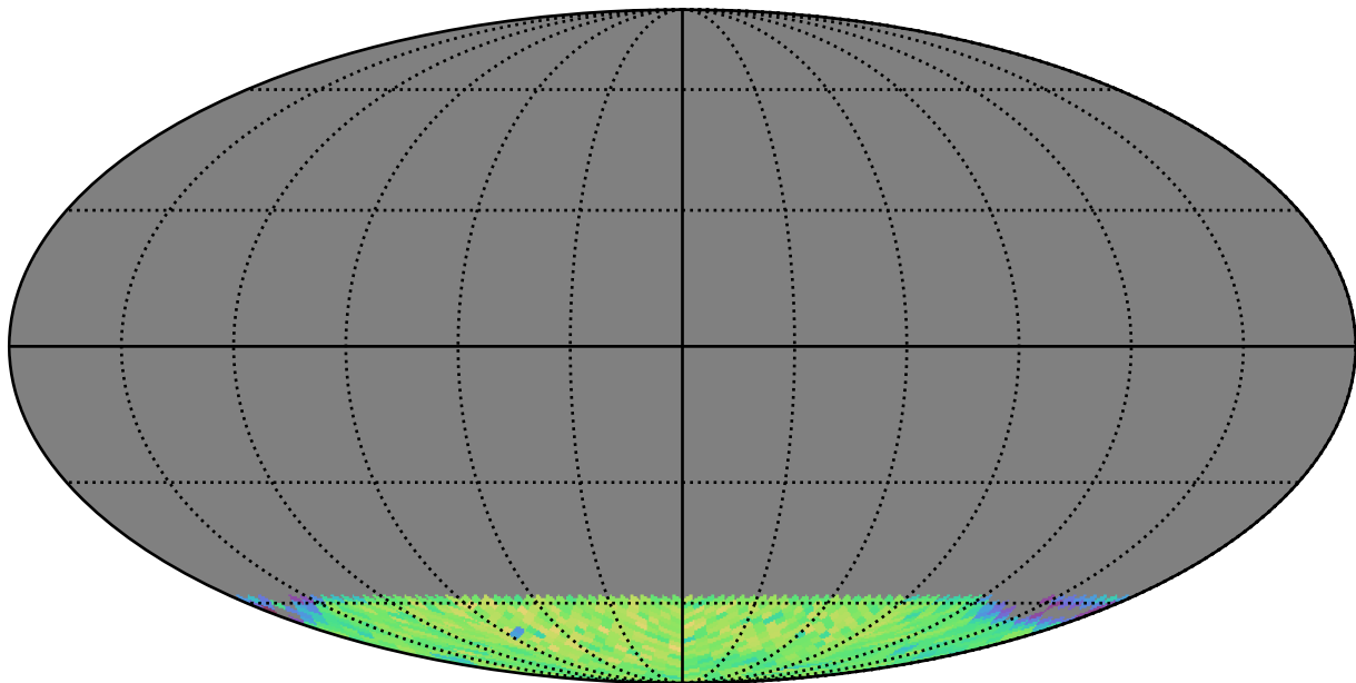
weather_cloudso2v3.5_10yrs gi SCP: LVDwarfs
