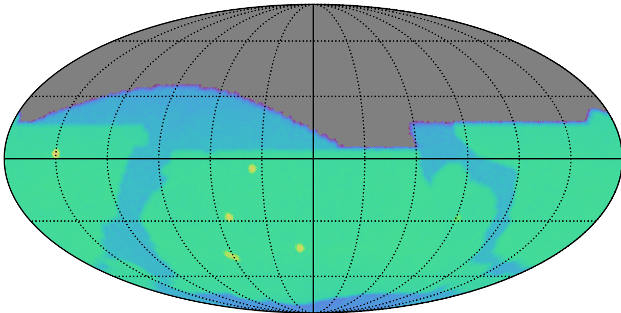
weather_cloudso2v3.5_10yrs i: SurfaceBrightLimit
