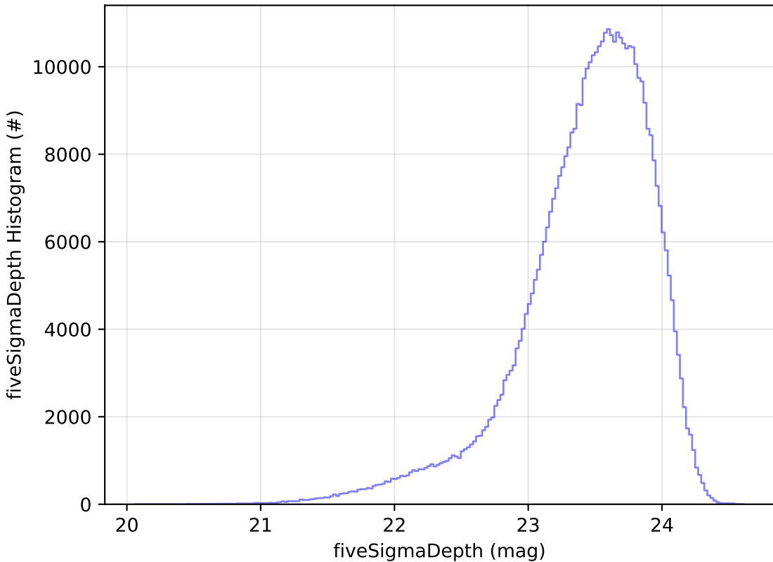
weather_cloudso2v3.5_10yrs i: fiveSigmaDepth Histogram
