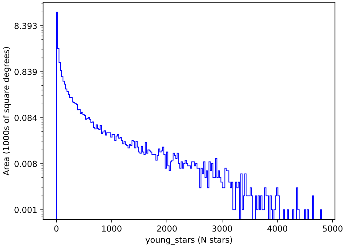
weather_cloudso2v3.5_10yrs : young_stars
