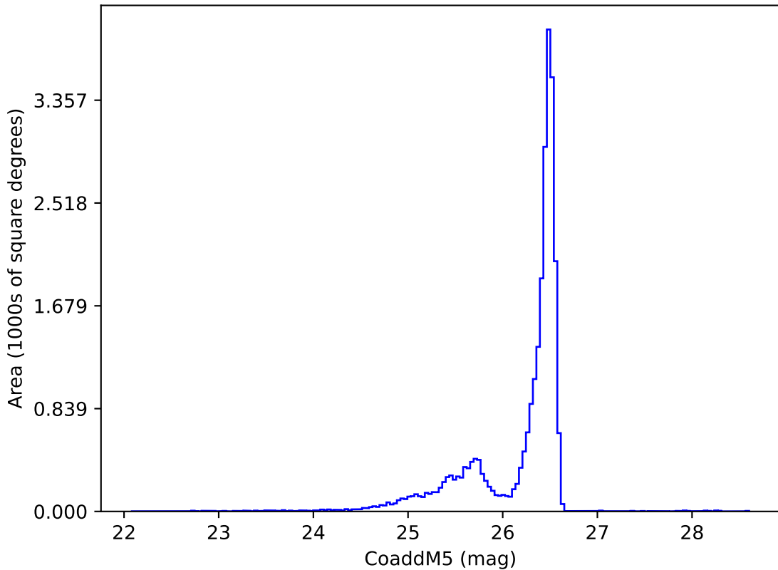
weather_cloudso31v3.5_10yrs i: CoaddM5
