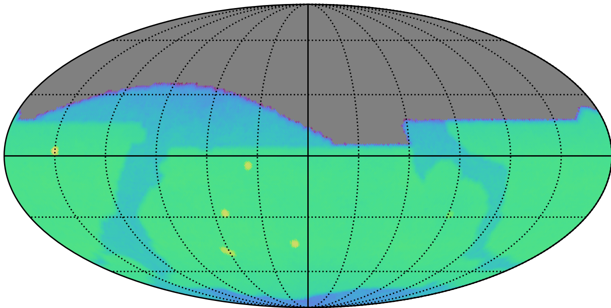
weather_cloudso31v3.5_10yrs i: CoaddM5
