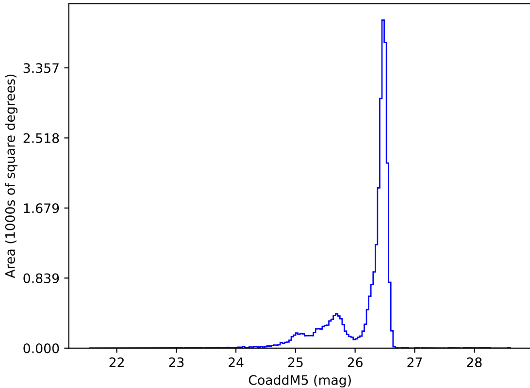
weather_cloudso35v3.5_10yrs i: CoaddM5
