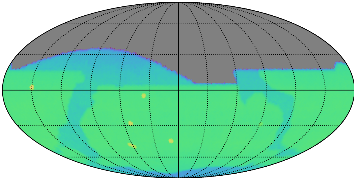
weather_cloudso35v3.5_10yrs i: CoaddM5
